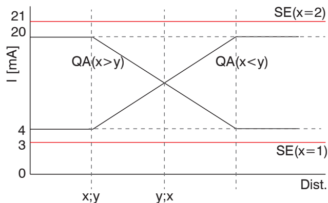
Fig. 20 Analog output
