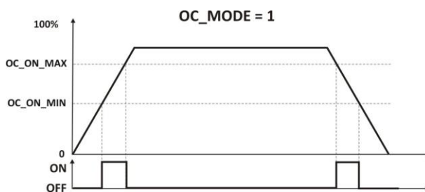
Rys. 5 Tryb pracy wyjścia OC_MODE =1
