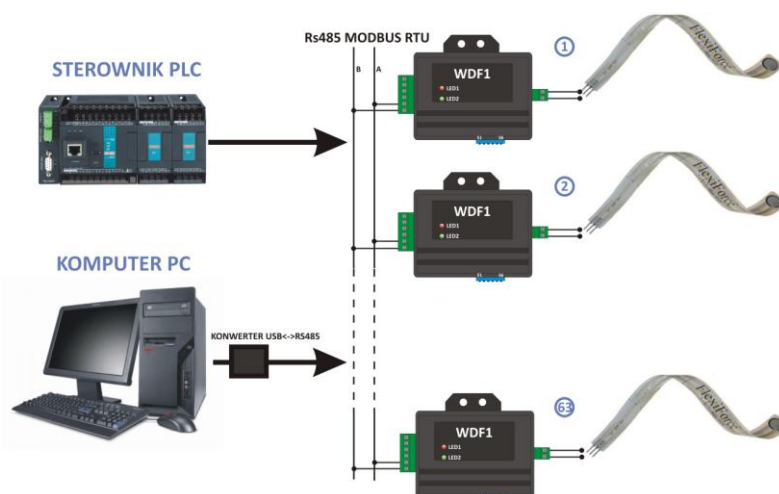
Rys. 7 Połączenie na magistrali MODBUS
