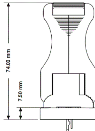
Paddle option „1“
